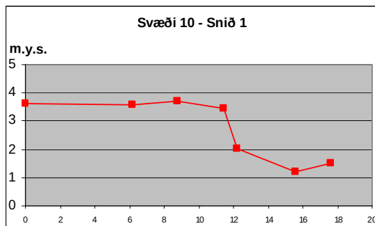
12. Mynd, svæði 10 Mældir punktar á bakka og í sniðum.
