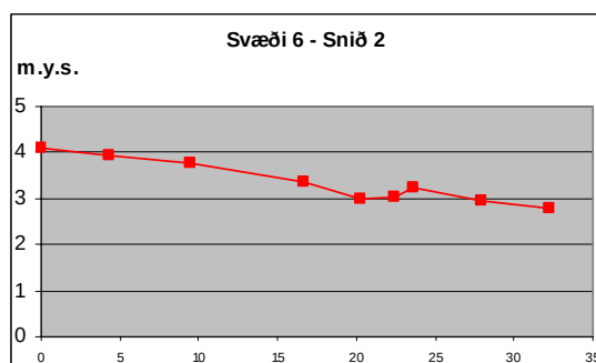
8. Mynd, svæði 6 Mældir punktar á bakka og í sniðum.
