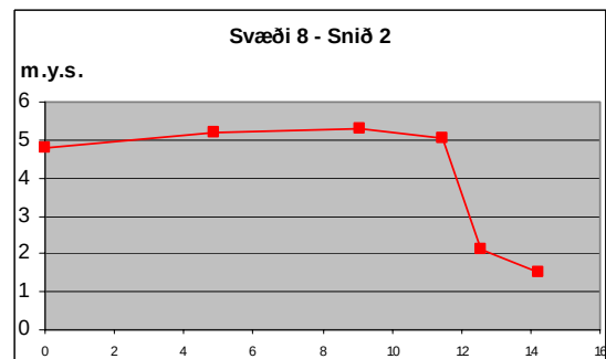
10. Mynd, svæði 8 Mældir punktar á bakka og í sniðum.
