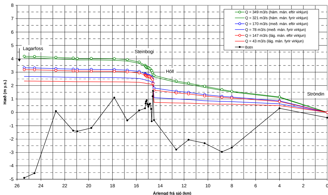
1. Mynd: Vatnsborðshæð í Lagarfljóti neðan Lagarfoss, fyrir og eftir tilkomu Kárahnjúkavirkjunar við meðalrennsli í vatnsmesta mánuði ársins (júní), meðalmánuði og vatnsminnsta mánuði ársins (janúar).
