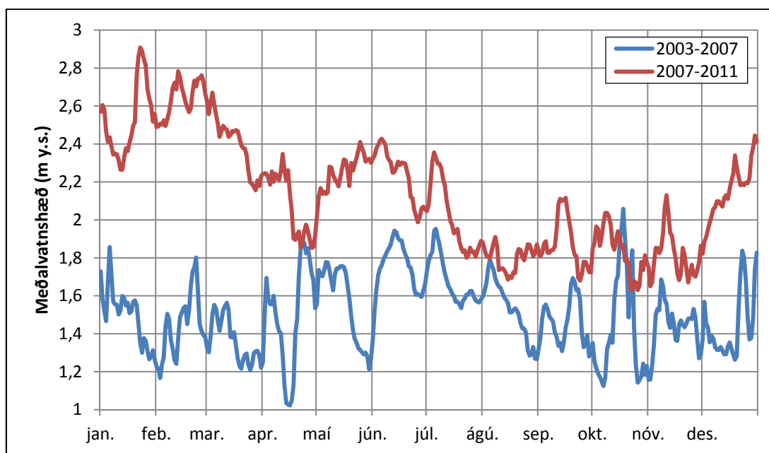
Mynd 15. Meðalvatnshæð Lagarfljóts við Hól V434 áráðilin 2003–2007 og 2007–2011.
