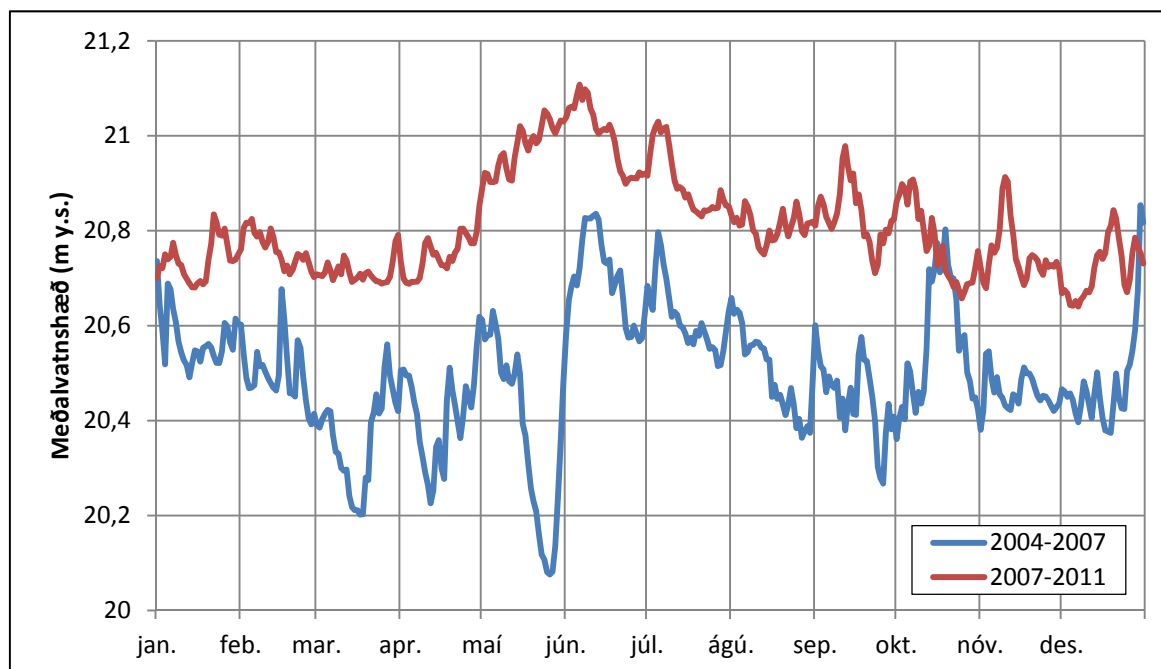
Mynd 9. Meðalvatnshæð Jökulsár í Fljótssdal við nýju brúna við Hólma V396 árabílin 2004–2007 og 2007–2011.
