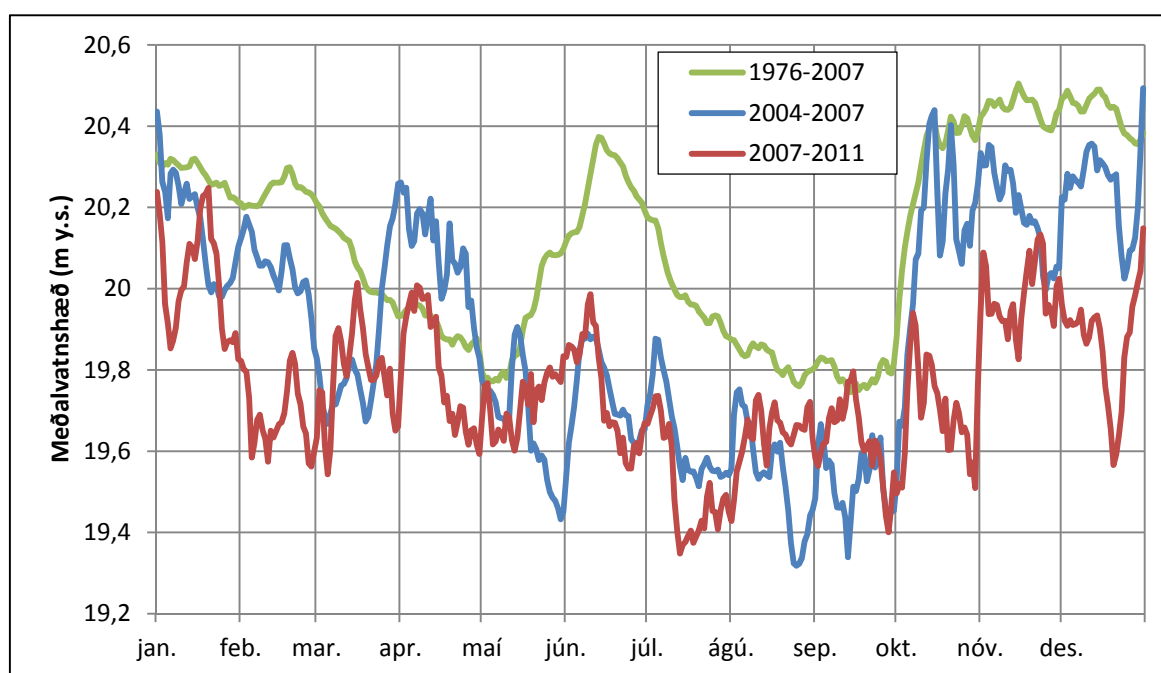
Mynd 14. Meðalvatnshæð við Lagarfoss V17 árábilin 1976–2007, 2004–2007 og 2007–2011.
