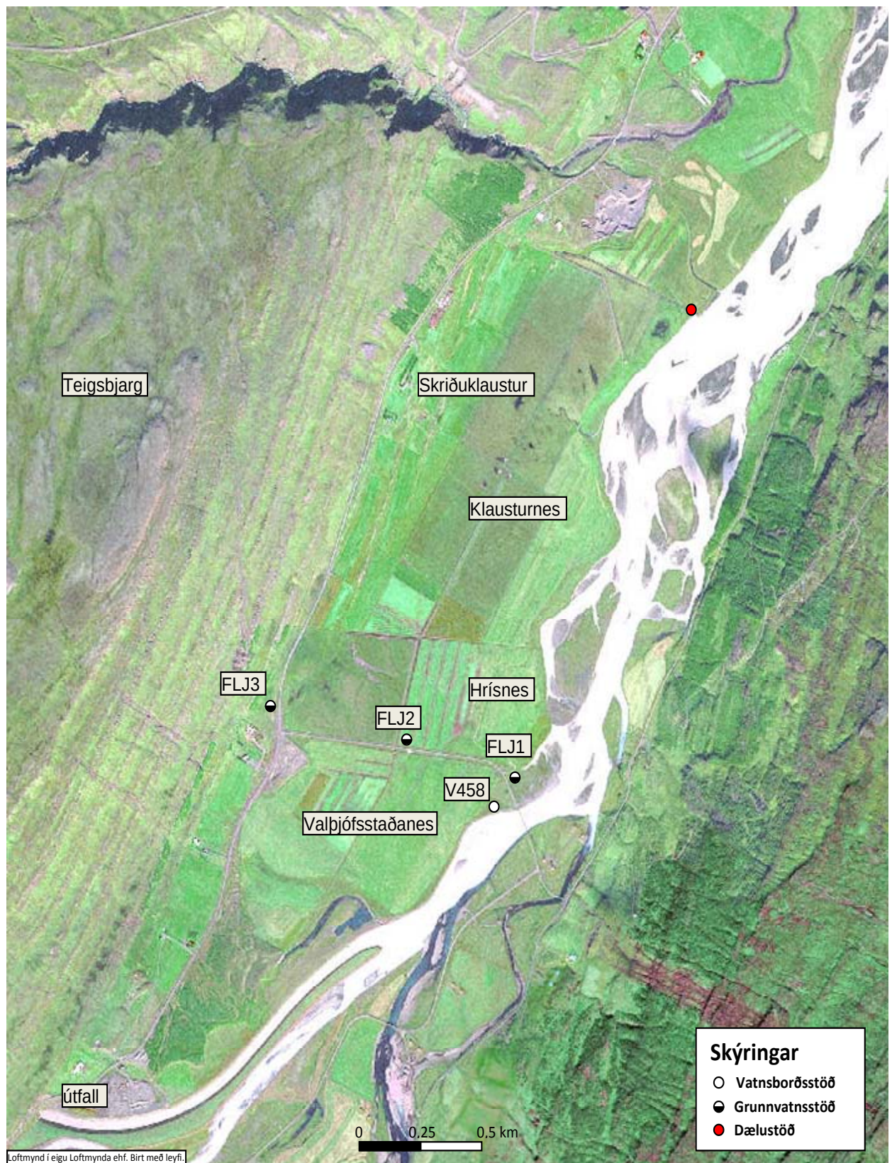
Mynd 2. Mælakerfi vegna vöktunar á grunnvatns- og vatnsborði í Fljótisdal.
