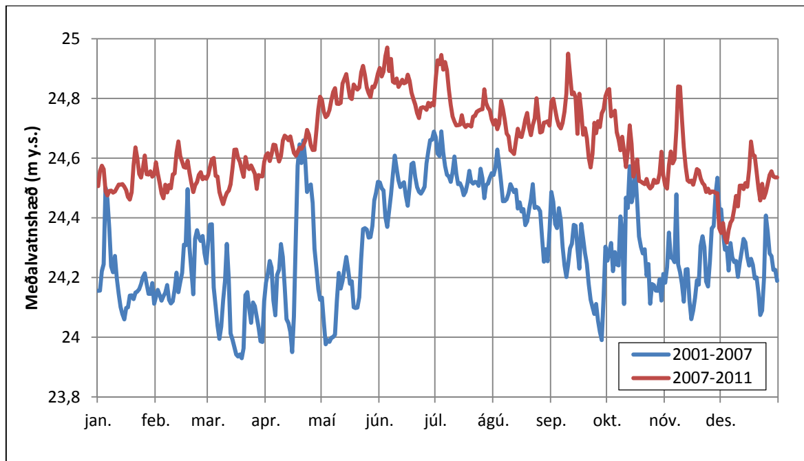
Mynd 3. Meðalvatnshæð Jökulsár í Fljótsdal við Valþjófsstaðarnes V458 árábilin 2001–2007 og 2007–2011.
