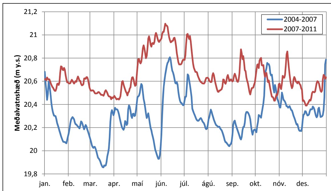
Mynd 10. Meðalvatnshæð Lagarfljóts við Buðlungavelli V397 árablin 2004–2007 og 2007–2011.
