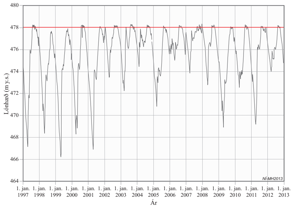
3. mynd. Vatnsborð Blöndulóns 1997-2012, mælt með sírita í Blöndustíflu. (Gögn frá Landsvirkjun).
