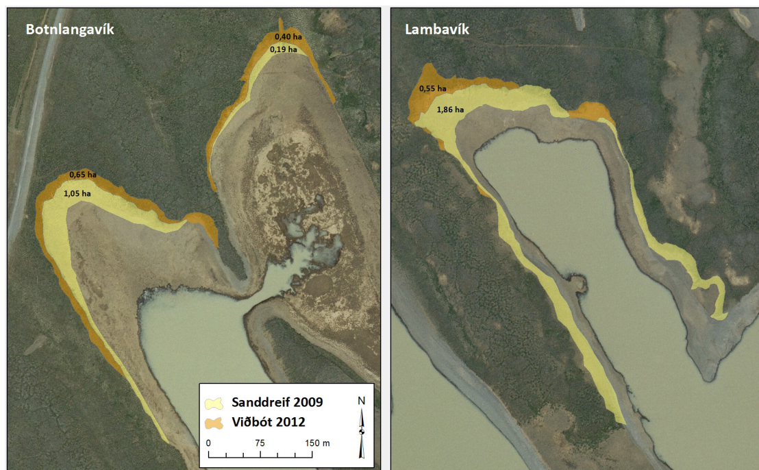
8. mynd. Útbreiðsla sands fyrir botni Lambavíkur og Botnlangavíkur haustið 2012. Loftmynd frá 21. júlí 2010, lónhæð 476,27 m eða tæpum 2 m undir yfirfallshæð. Jaðar sanddreifar 2009 markar stöðu lónborðs við yfirfall. Lagt er til að girt verði fyrir botn Lambavíkur og vesturhluta Botnlangavíkur vorið 2013 til að friða fyrir beit, auðvelda uppgræðslu og heftingu sandfoks.
