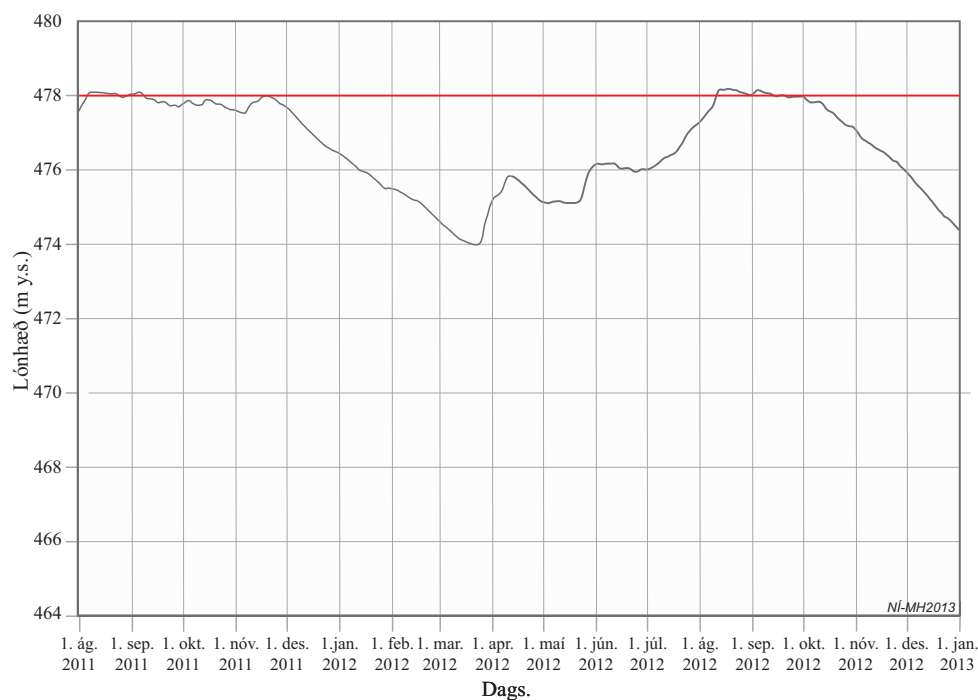
2. mynd. Vatnsborð Blöndulóns frá 1. ágúst 2011 til ársloka 2012, mælt með sírta í Blöndustíflu. Yfirfall, 478,0 m, er merkt með rauðri línu. (Gögn frá Landsvirkjun, Wiski gagnagrunnur, 2013.01.10.).
