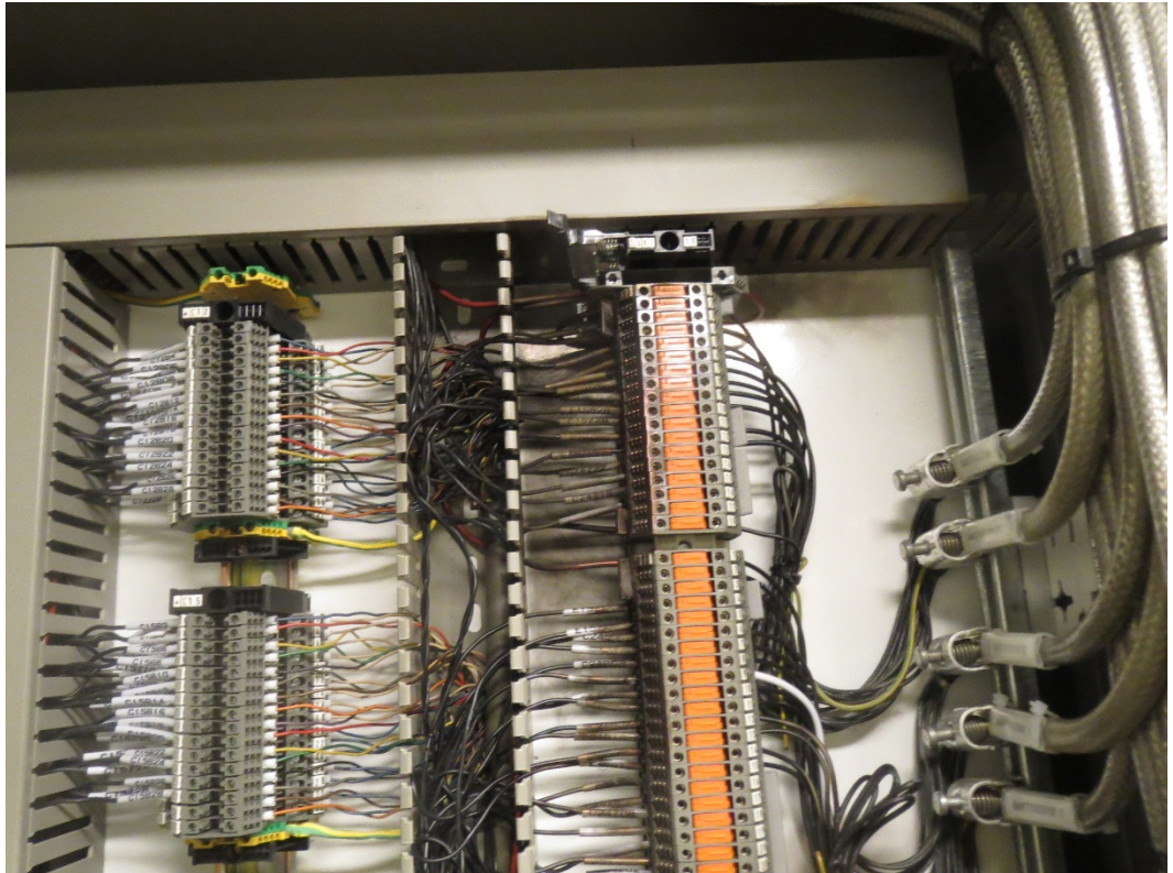
Afleiðing yfirspennu í rafmagnsskáp þegar háspennuskot kom inn á jafnstraumskerfi í Kröfluvirkjun
