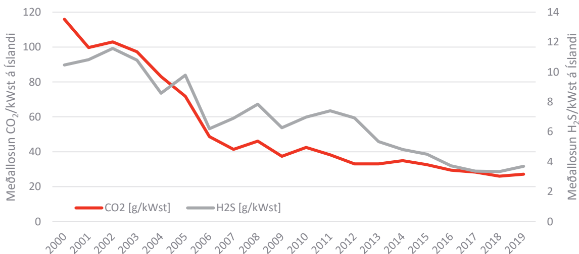
MYND 27 Meðallosun CO 2 og H 2 S á hverja framleidda kílóvattstund frá jarðvarmavirkjunum á Íslandi sem vinna rafmagn 2000-2018. Talnaefni Orkustofnunar, OS-2020-T002-01 (2020) [10].
