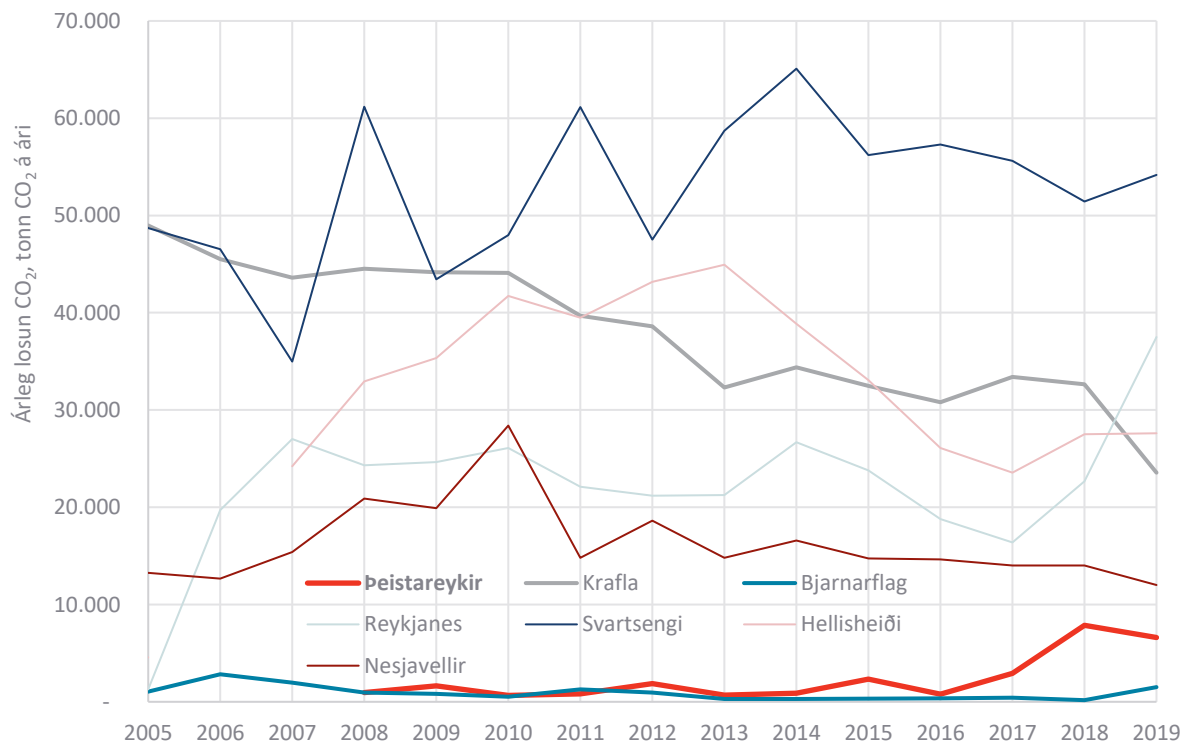
MYND 29 Árlæg heildarlosun koltvísýrings frá íslenskum jarðvarmavirkjunum. Stöðvarnar vinna ýmist eingöngu raforku eða bæði raforku og heitt vatn. Talnaefni Orkustofnunar, OS-2020-T002-01 (2020) [10].
