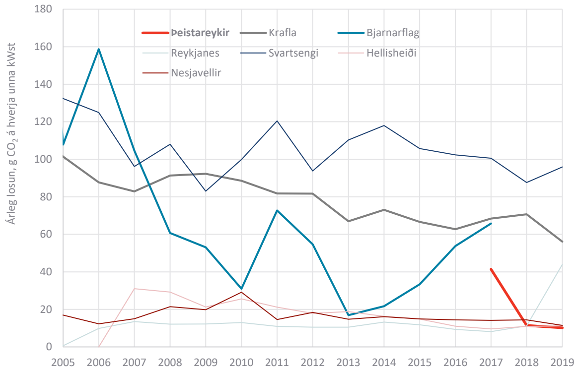
MYND 28 Árlæg losun koltvísýrings frá íslenskum jarðvarmavirkjunum á hverja framleidda kílóvattstund (kWst) af rafmagni. Talnaefni Orkustofnunar, OS-2020-T002-01 (2020) [10].
