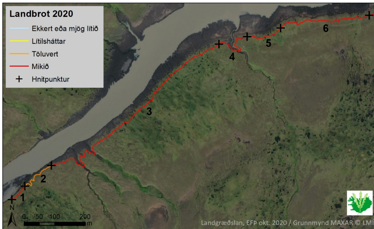
Kort 3. Landbrot við Kringilsá skv. úttekt sumarið 2020.
