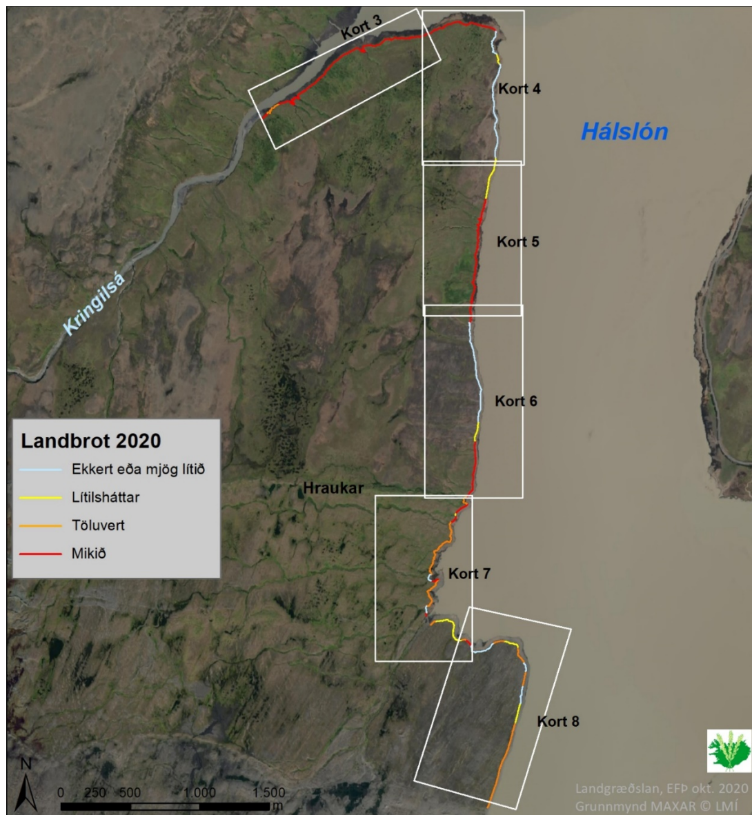
Kort 2. Heildaryfirlit yfir landbrot í Kringilsárrana skv. úttekt sumarið 2020. Hvítir rammar og númer vísa til korta í þessari skýrslu þar sem nánar er gerð grein fyrir landbroti einstakra svæða.
