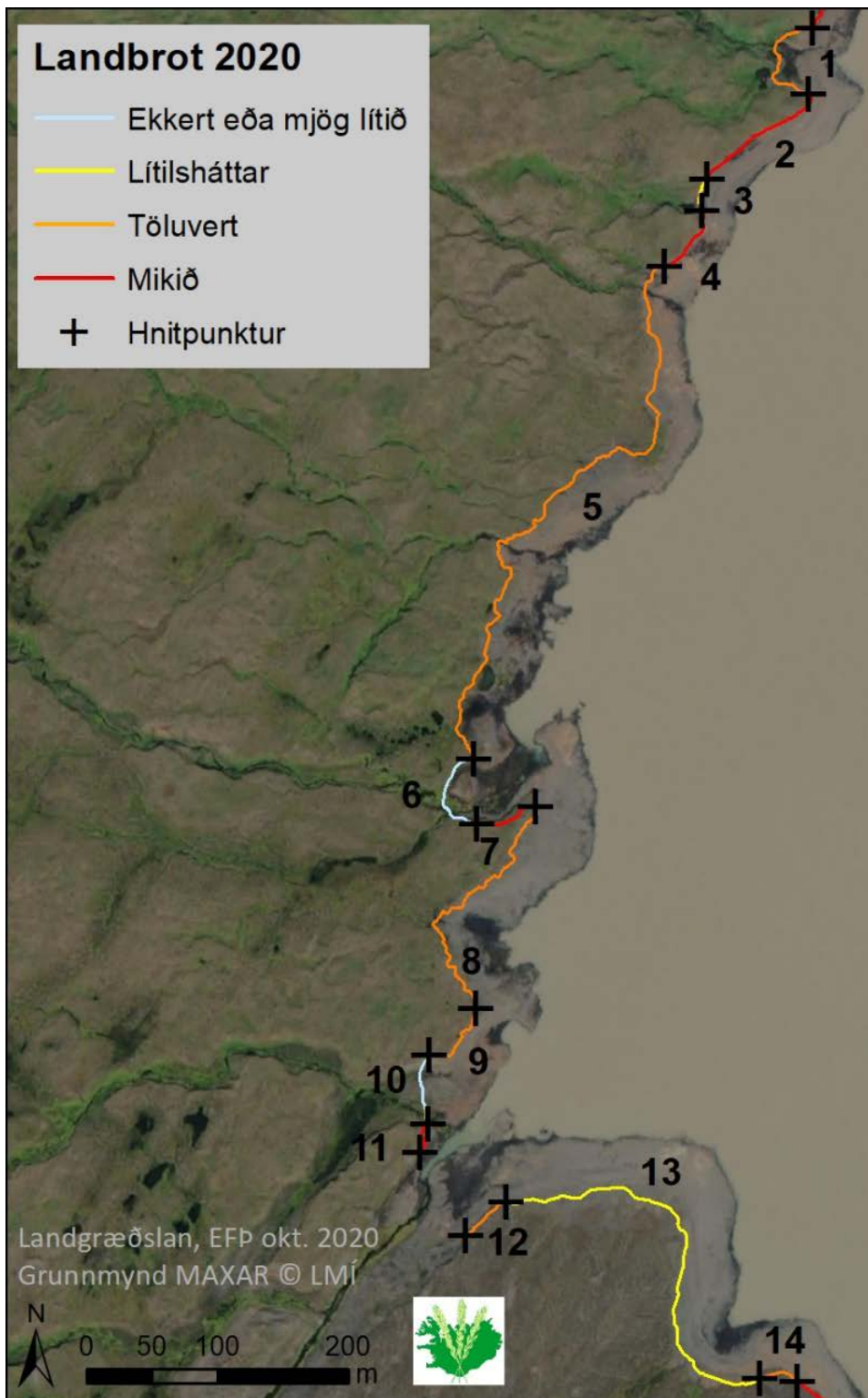
Kort 7. Landbrot við austurströnd Kringilsárrana sunnan Hrauka skv. úttekt sumarið 2020.
